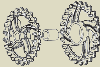
Crossskill ø480 mm/530 mm und Crossskill HD ø550/600 mm (bei Actiroll HD)
